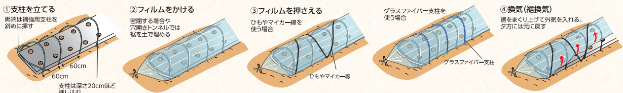
図 トンネルの作り方
